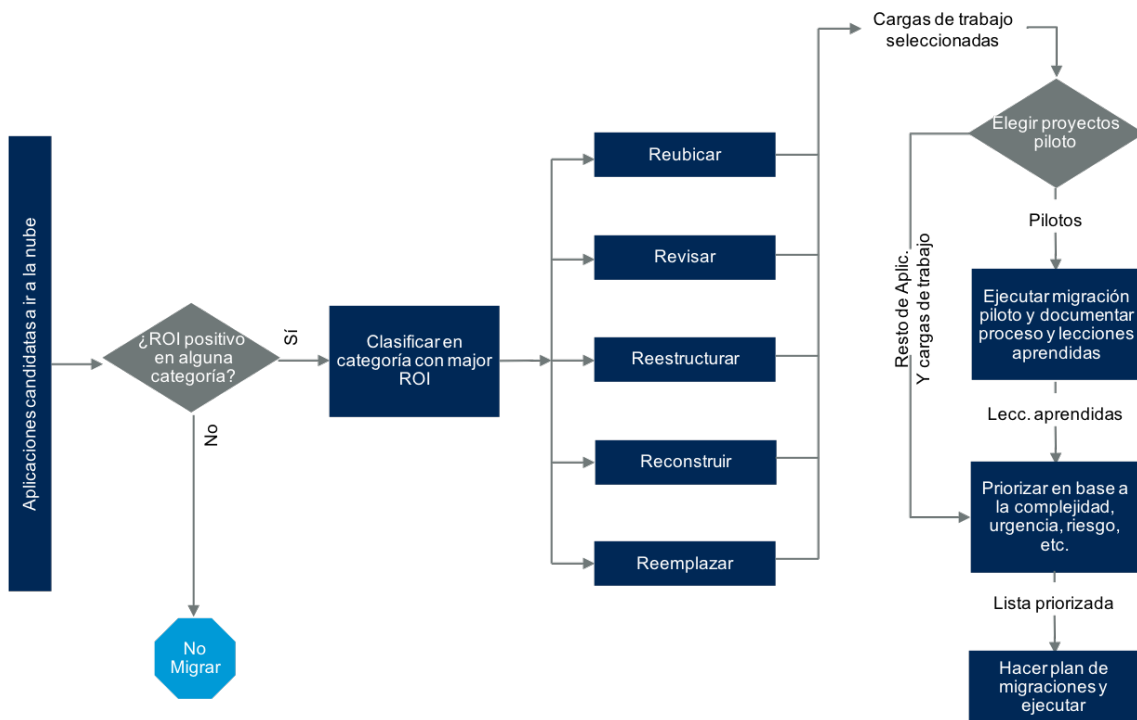
Figura 5. Diagrama de flujo para la migración de aplicaciones a la nube
